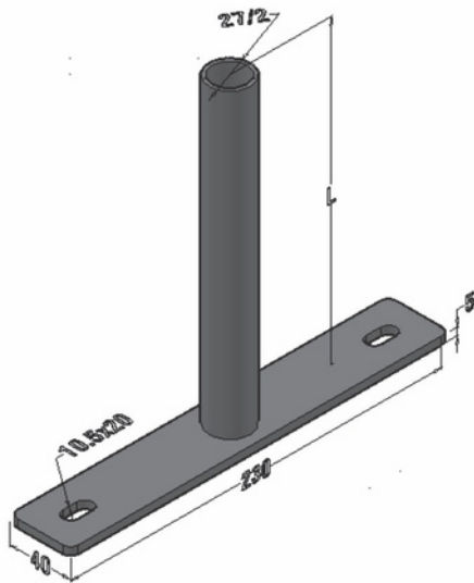
HARİCİ BORU DİREĞİ EXTERIOR PIPE FOOT
