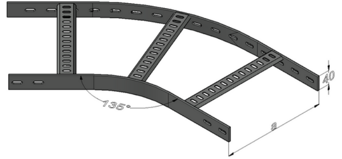
45° DELİKLİ TİP KABLO MERDİVENİ DÖNÜŞ ELEMANLARI 45° PERFORATED CABLE LADDER TURNS
