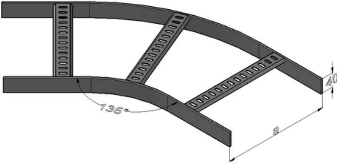
45 KABLO MERDİVENİ DÖNÜŞ ELEMANLARI 45 CABLE LADDER TURNING ELEMENTS
