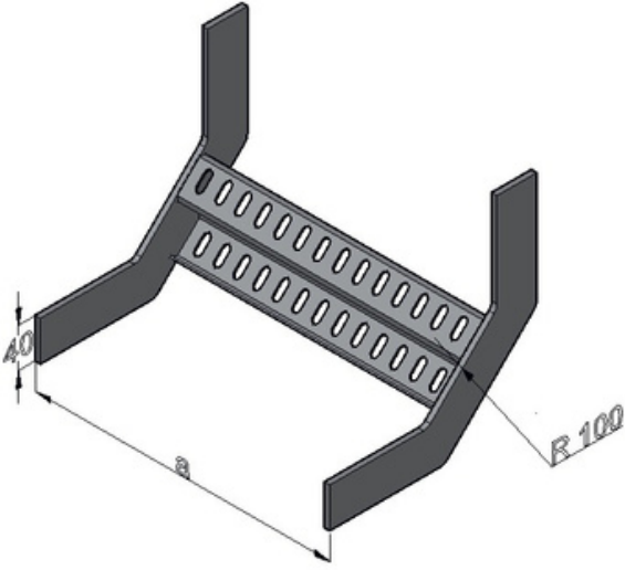
SİMETRİK İÇ BÜKEY ELEMANLARI SYMMETRICAL TYPE INSIDE ELBOWS
